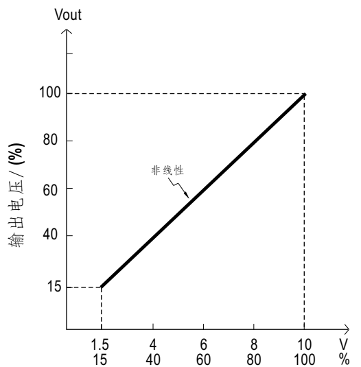
PIN5/PIN6接入的外部电压(DC)/PWM信号
