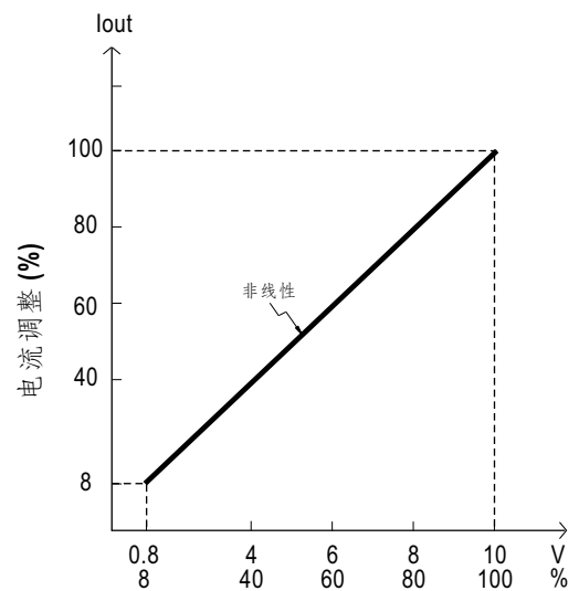
PIN5/PIN6接入的外部电压(DC)/PWM信号
